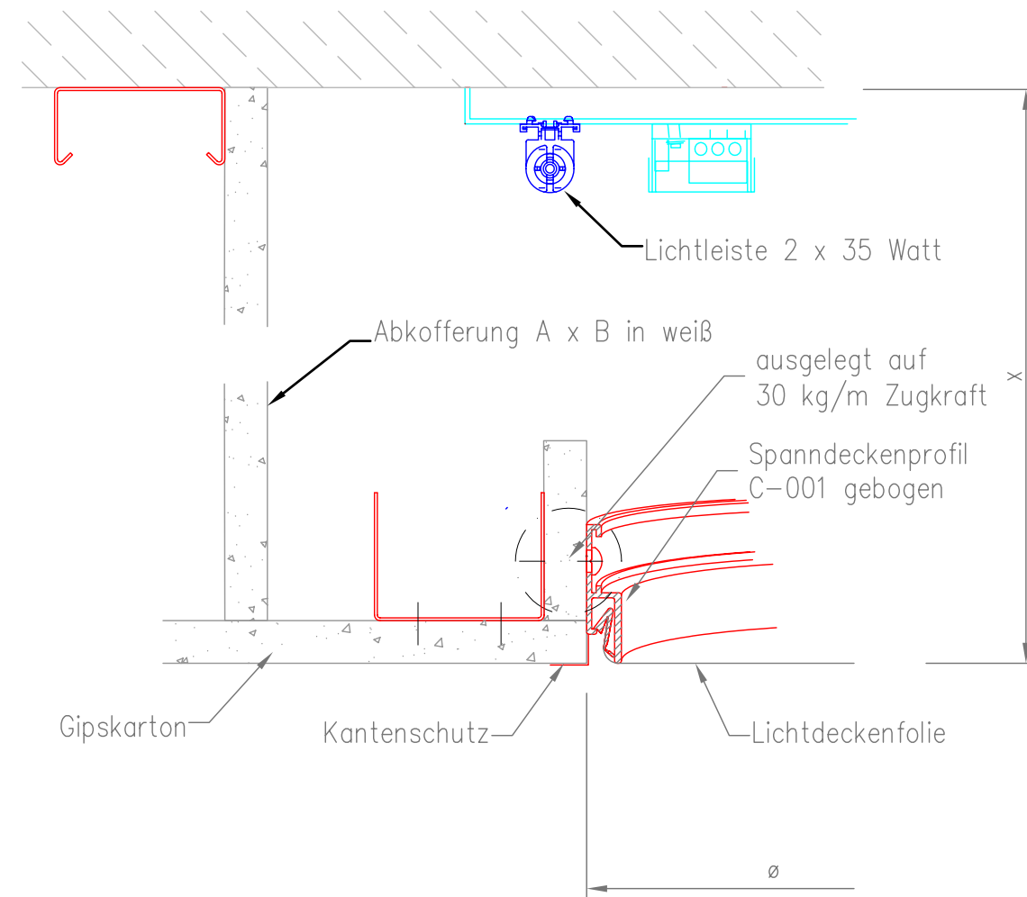
Schnitt A - A Maßstab 1:2
